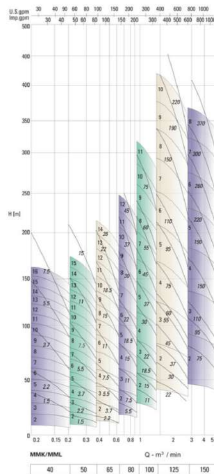
60Hz-4P (1800 r.p.m.)
