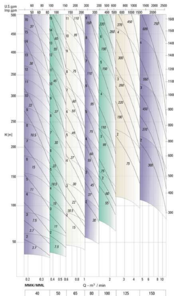
50Hz-2P (3000 r.p.m.)
