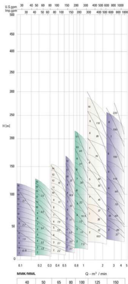
50Hz-4P (1500 r.p.m.)
