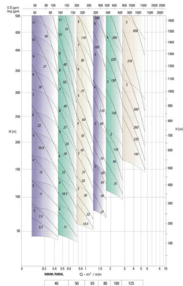
60Hz-2P (3600 r.p.m.)
