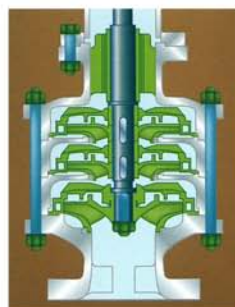
Radial impeller
